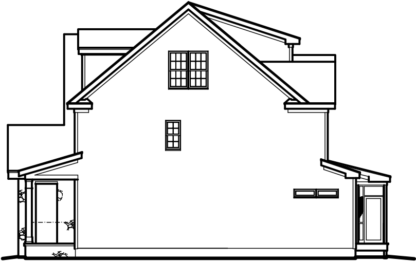
RIGHT ELEVATION
